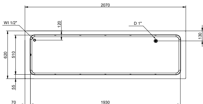
Boven aanzicht
